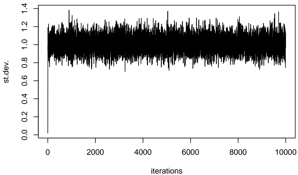
st.dev.
