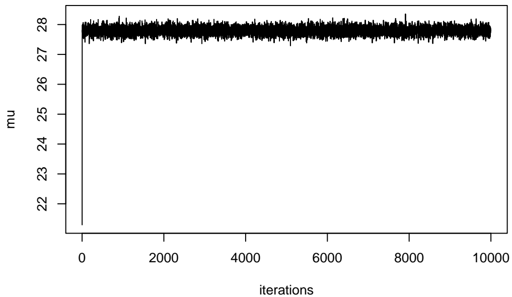
mu
